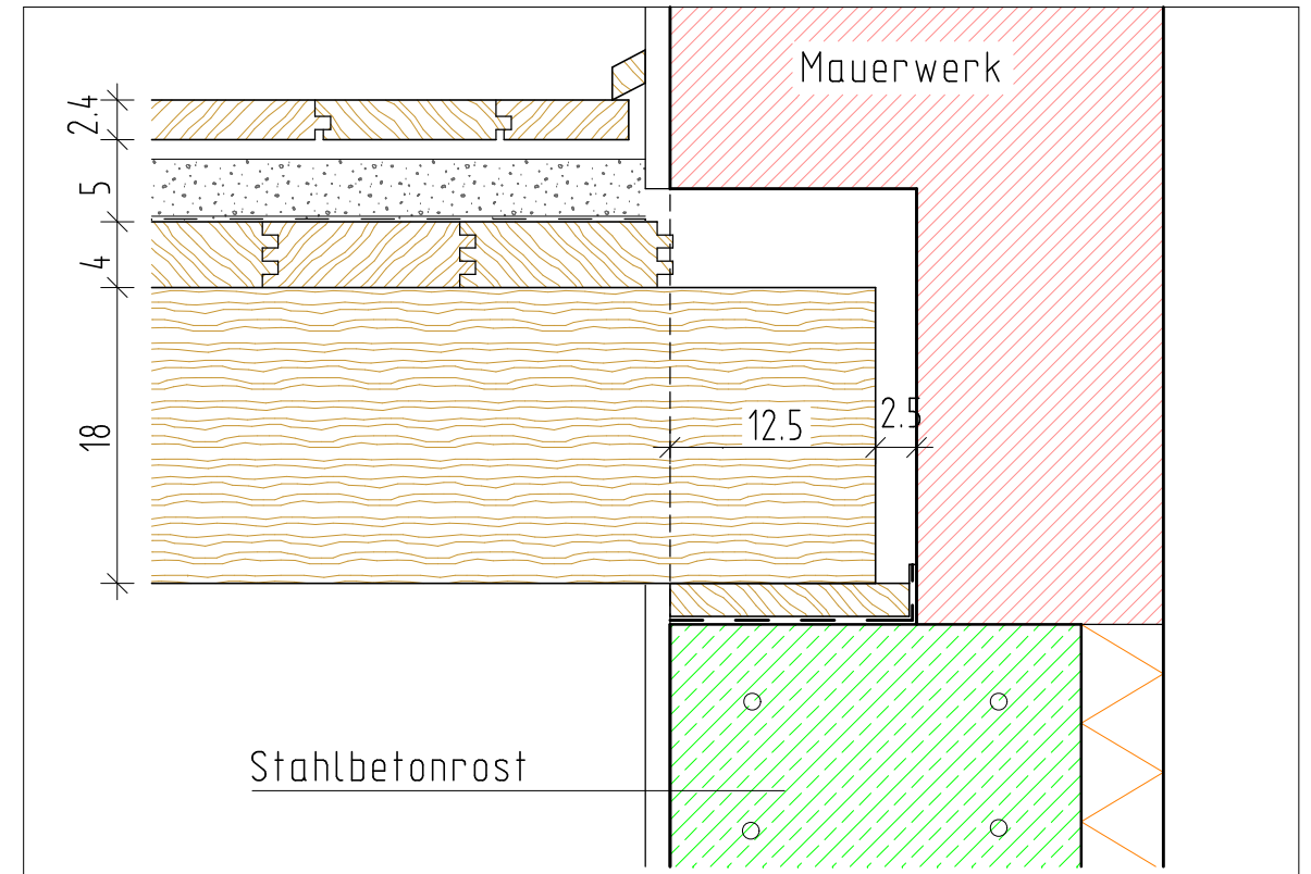
DECKENAUFBAU M 1:10
