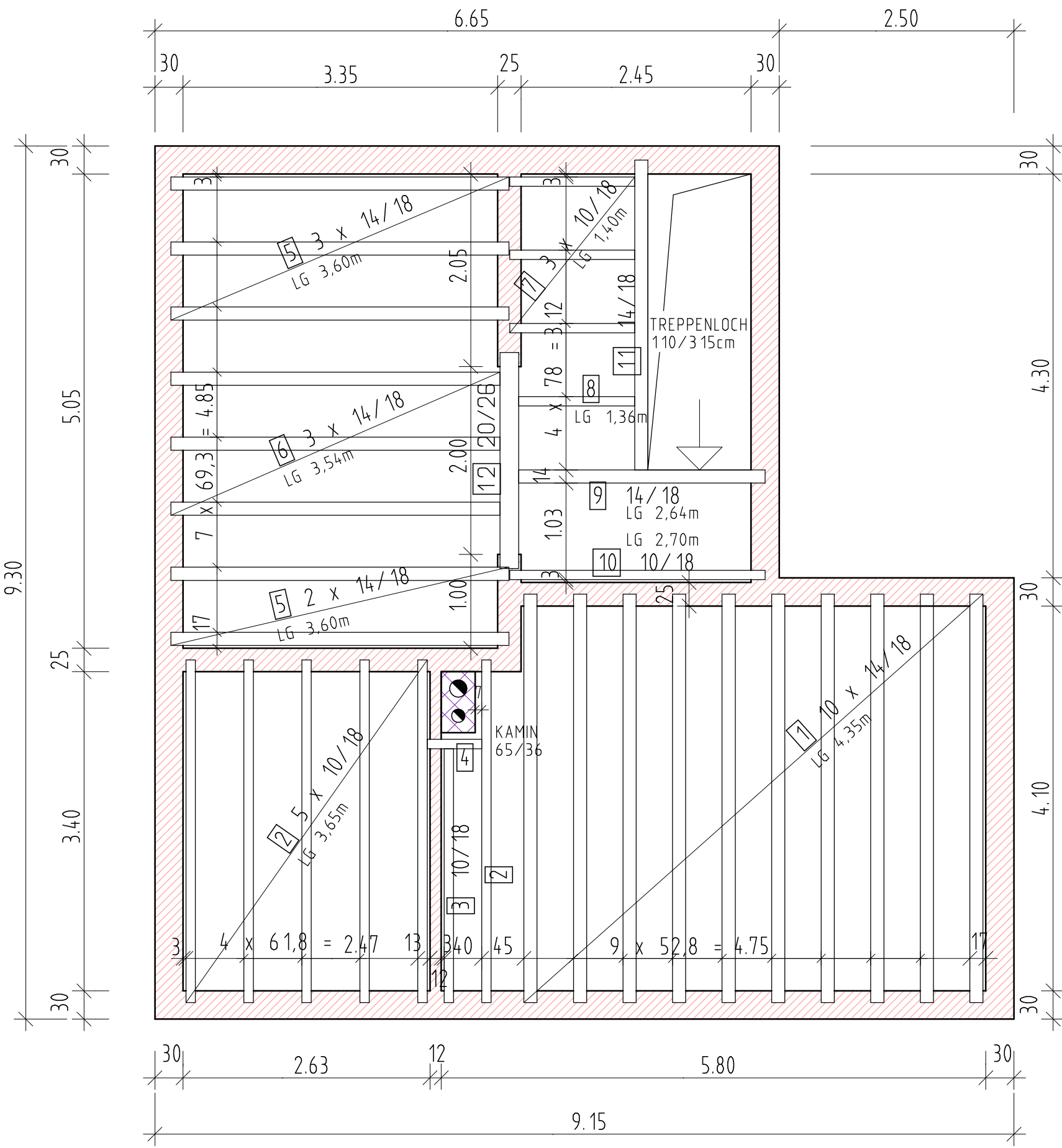
BALKENLAGE M 1:50
