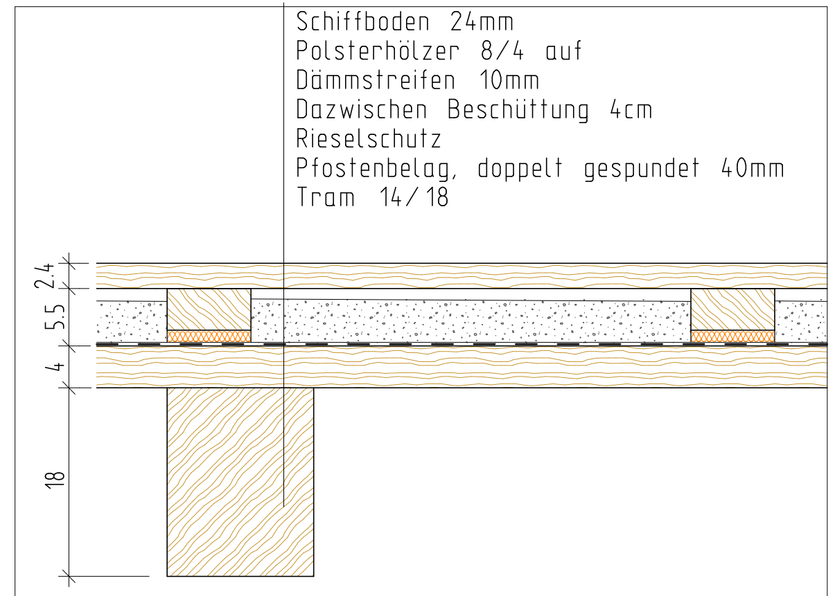
DECKENAUFBAU M 1:10
