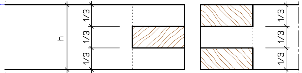
AUFRISS
