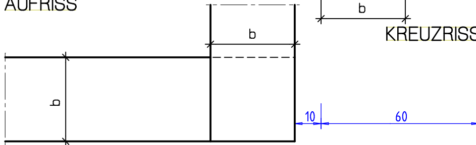
GRUNDRIS
